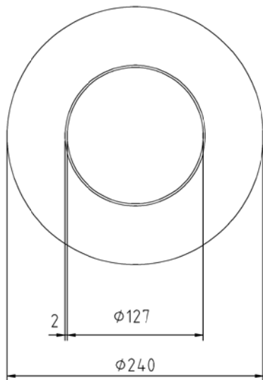
TOPP VY 1:5
