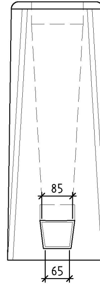
B-B 1:10
