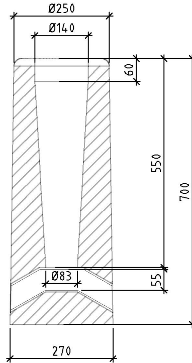
A-A 1:10
