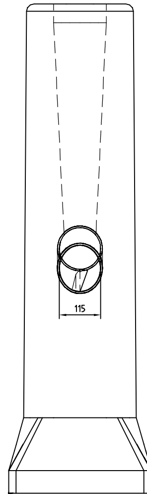
B-B 1:10
