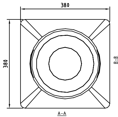
TOPP VY 1:10
