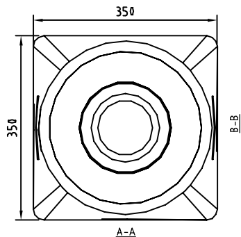
TOPP VY 1:10
