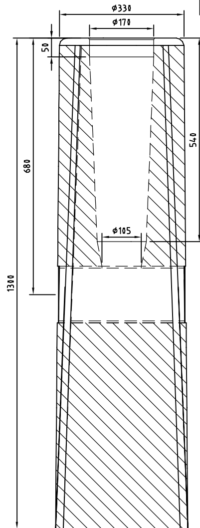
A-A 1:10
