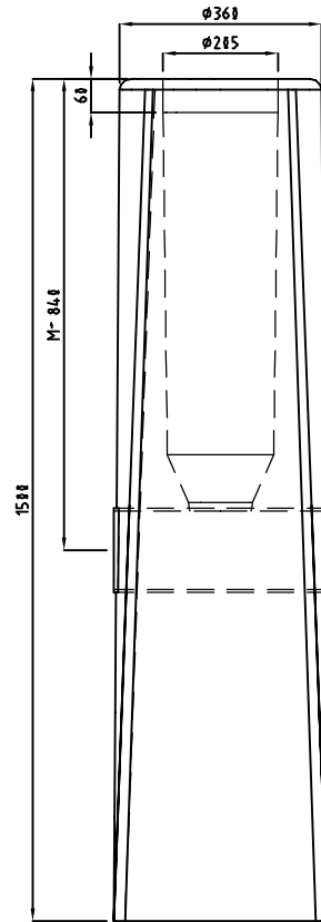
A-A 1:15
