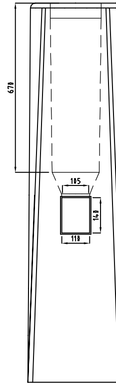
B-B 1:15
