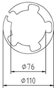
TOPP VY 1:5
