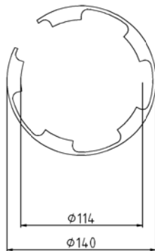
TOPP VY 1:5
