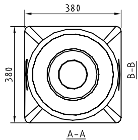
TOPP VY 1:15
