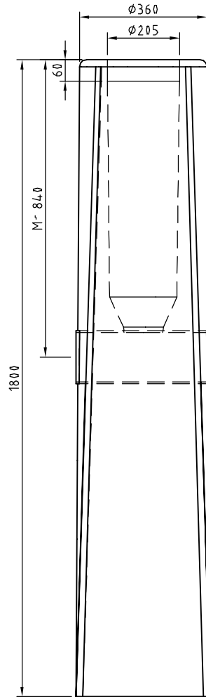
A-A 1:15
