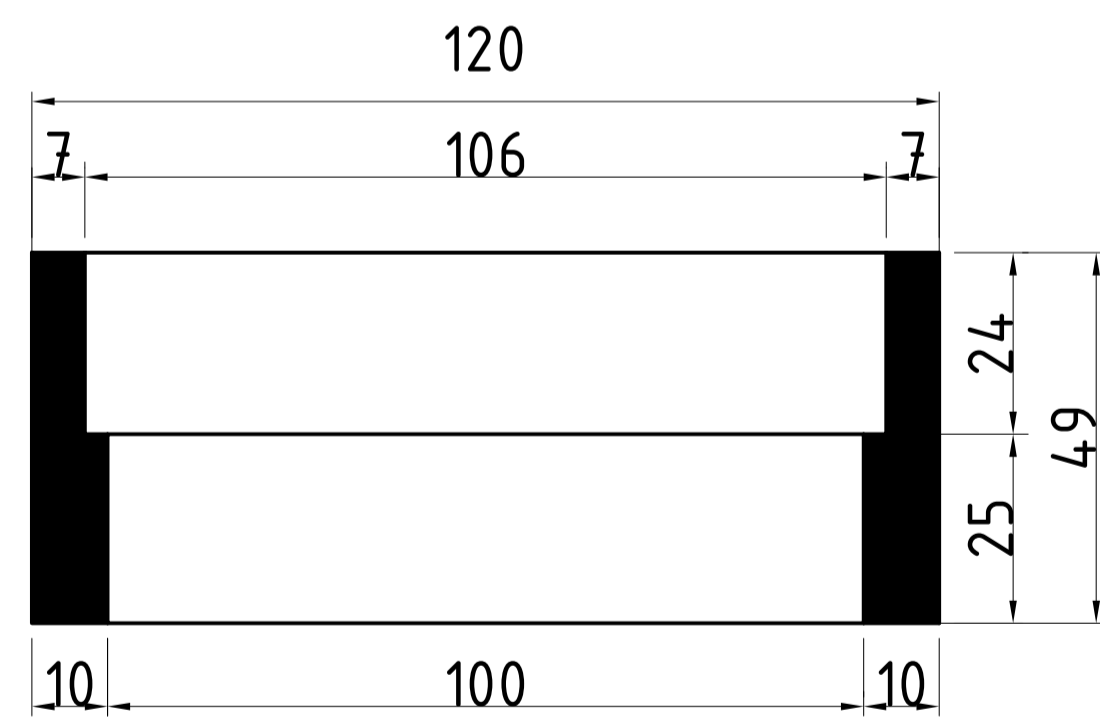
A-A 1:1
