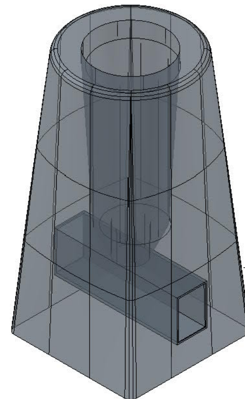
3D VY 1:10
