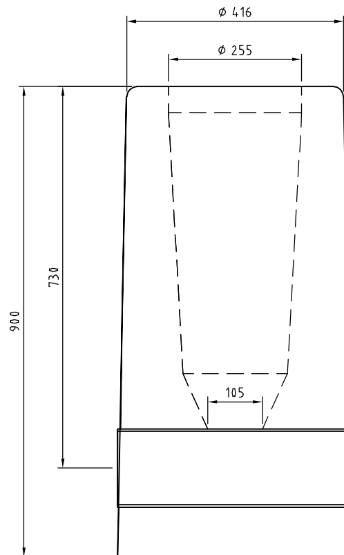
B-B 1:10
