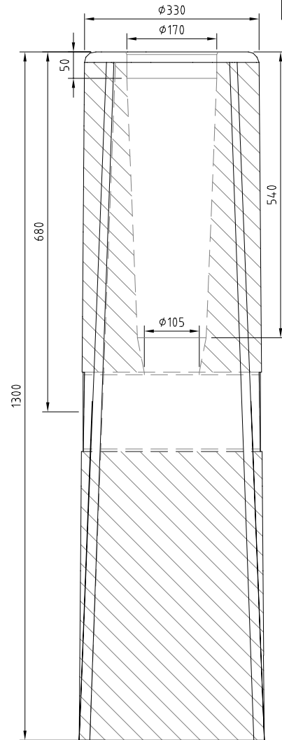
A-A 1:10
