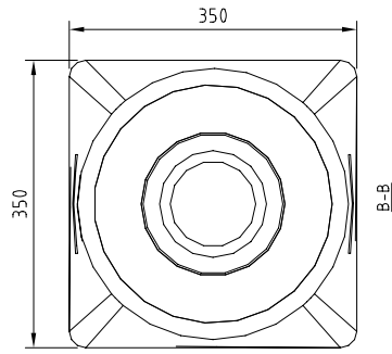
TOPP VY 1:10
