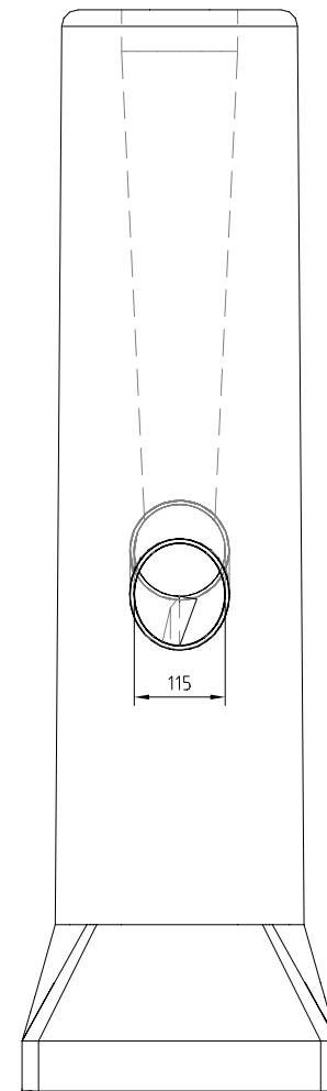
B-B 1:10
