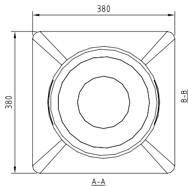
TOPP VY 1:10
