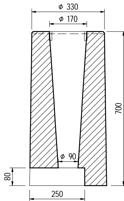
A-A 1 : 10
