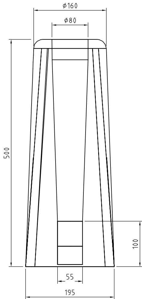
A-A 1:5
