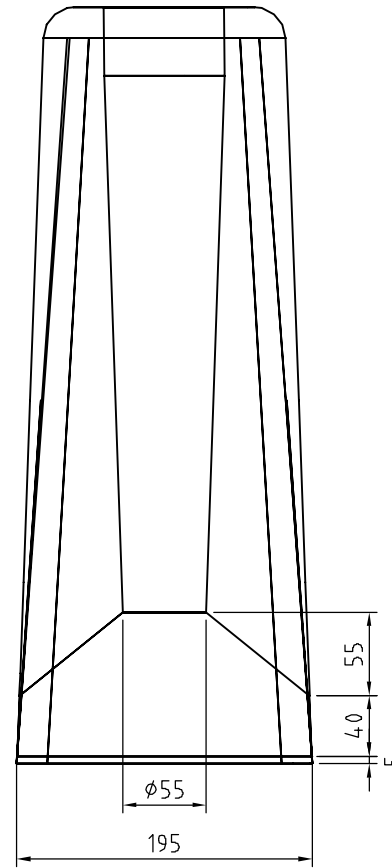
B-B 1:5
