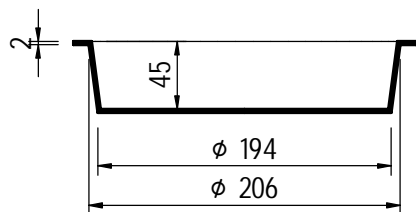
A-A 1 : 5
