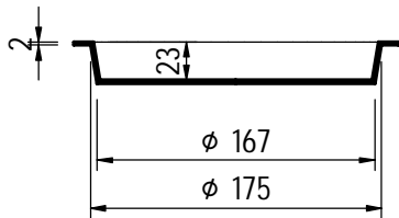
A-A 1 : 5
