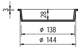
A-A 1 : 5
